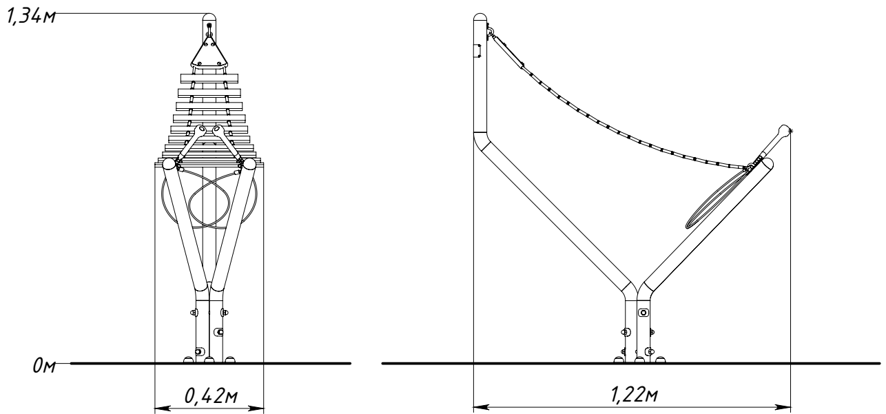
Рисунок 1 — Основные габаритные размеры
