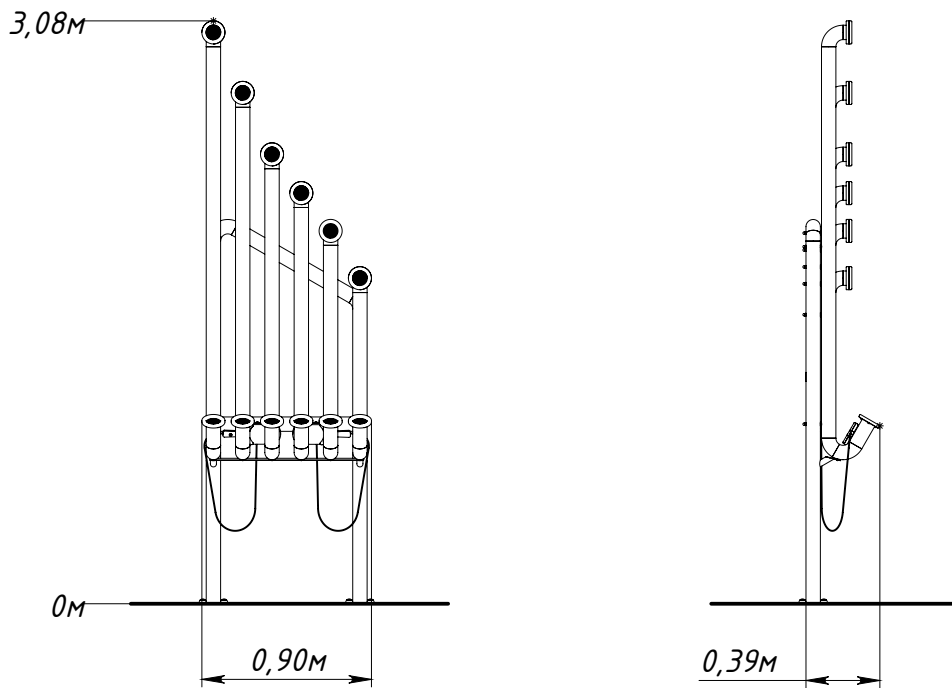
Рисунок 1 — Основные габаритные размеры
