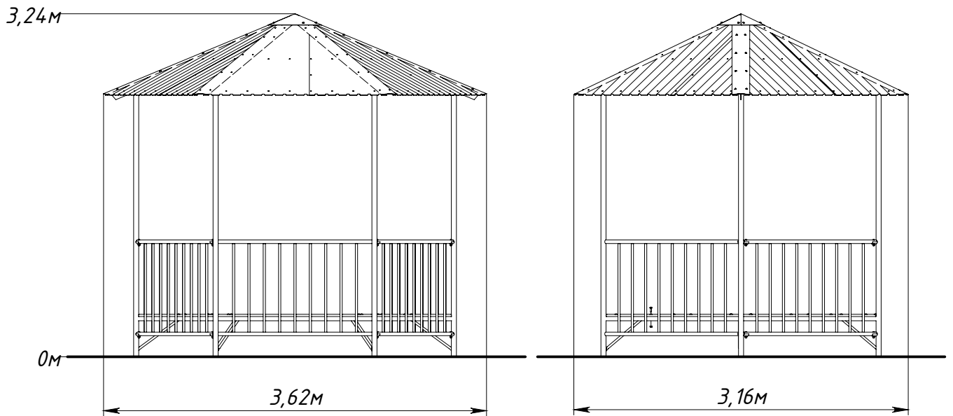
Рисунок 1 — Основные габаритные размеры
