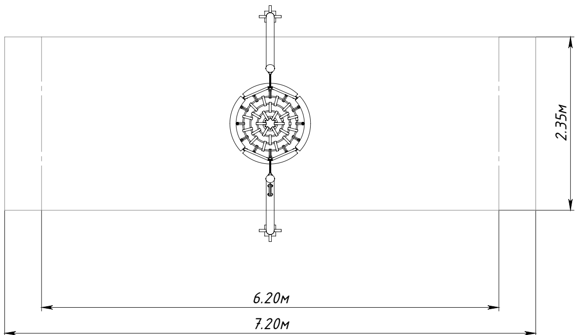
Рисунок 2 — Граница зоны приземления
